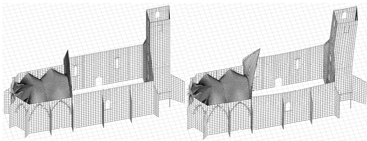
12. ábra – falazott szerkezetek mechanikai modellje: (a). a véges-elem rácsrendszer, (b). az egyik rezgésmód elmozdulásai
